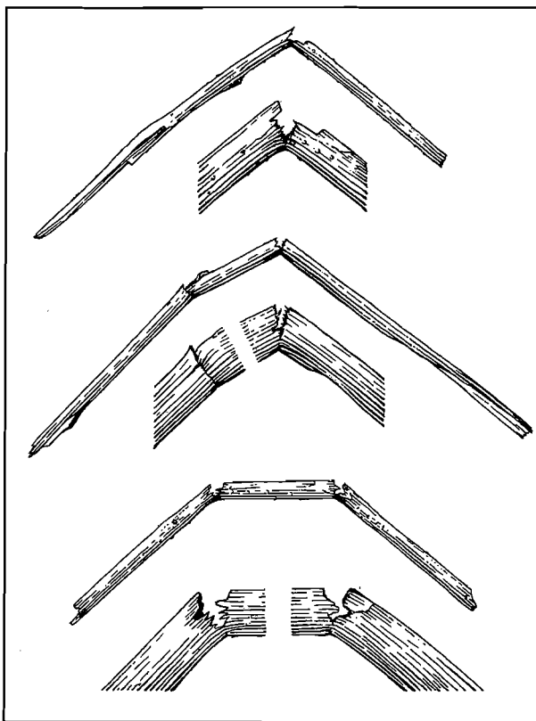
Abb. 2. Knickstäbe zum Ausreißen von Barthaar ( dela ), Holz der Trema tomentosa (L 19,5 cm, Ø 0,8 cm; L 21,5 cm, Ø 0,6 cm; L 17,0 cm, Ø 0,7 cm) — Imarin
