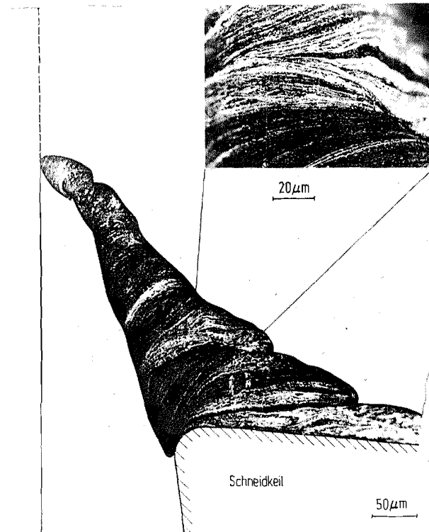
Abb. 3. Form und Struktur einer Aufbauschneide
