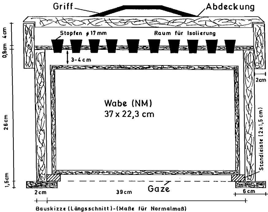
Abb. 4. Vorbrütkasten
